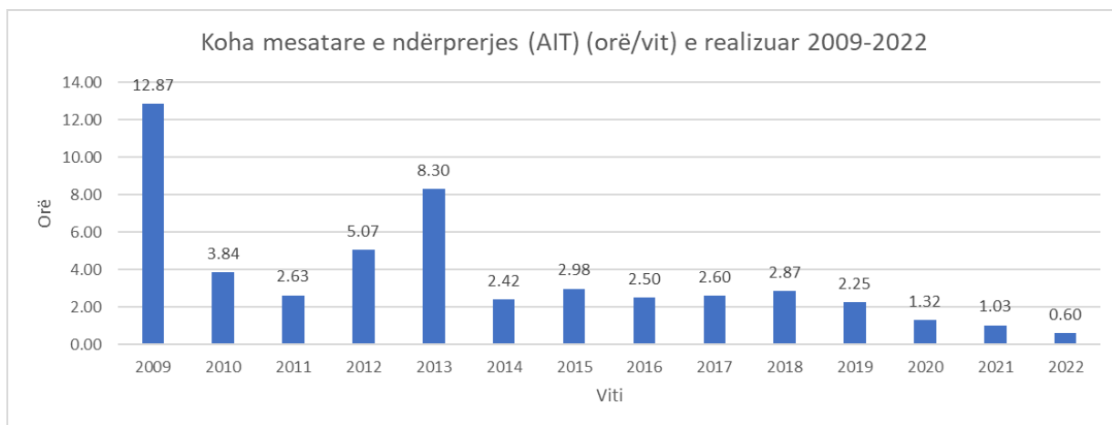
Figura 7-1. Koha mesatare e ndërprerjes vjetore të shkaktuar nga rrjeti transmetues përgjatë viteve paraprahe.
