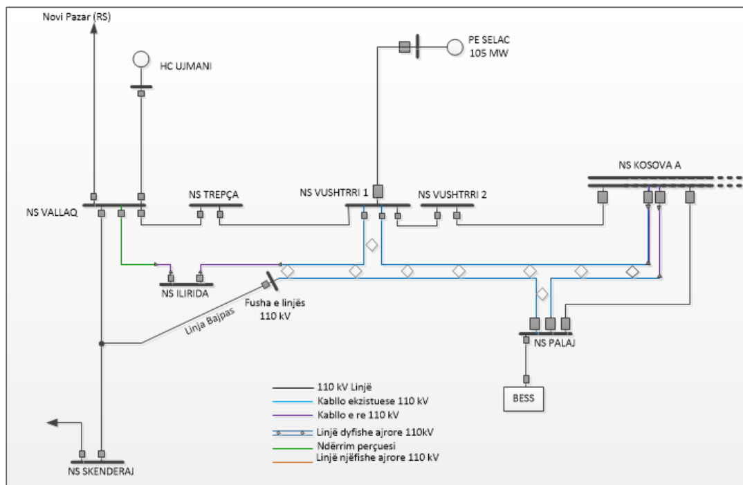
Figura 5-20 Skema njepolare e Projektit e Rivitalizimit te linjës NS Kosova A- NS Palaj- NS Ilirida-NS Vallaq
