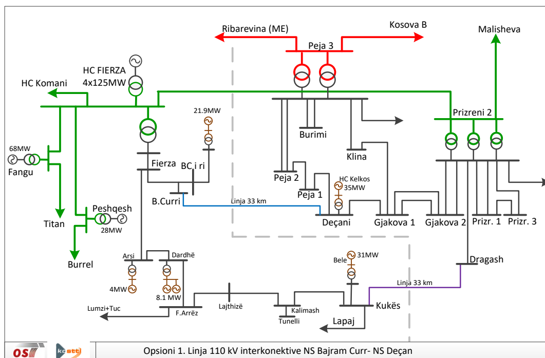
Figura 5-32. Projekti i linjës së dytë interkonektive NS Bajram Curri-NS Deçani
