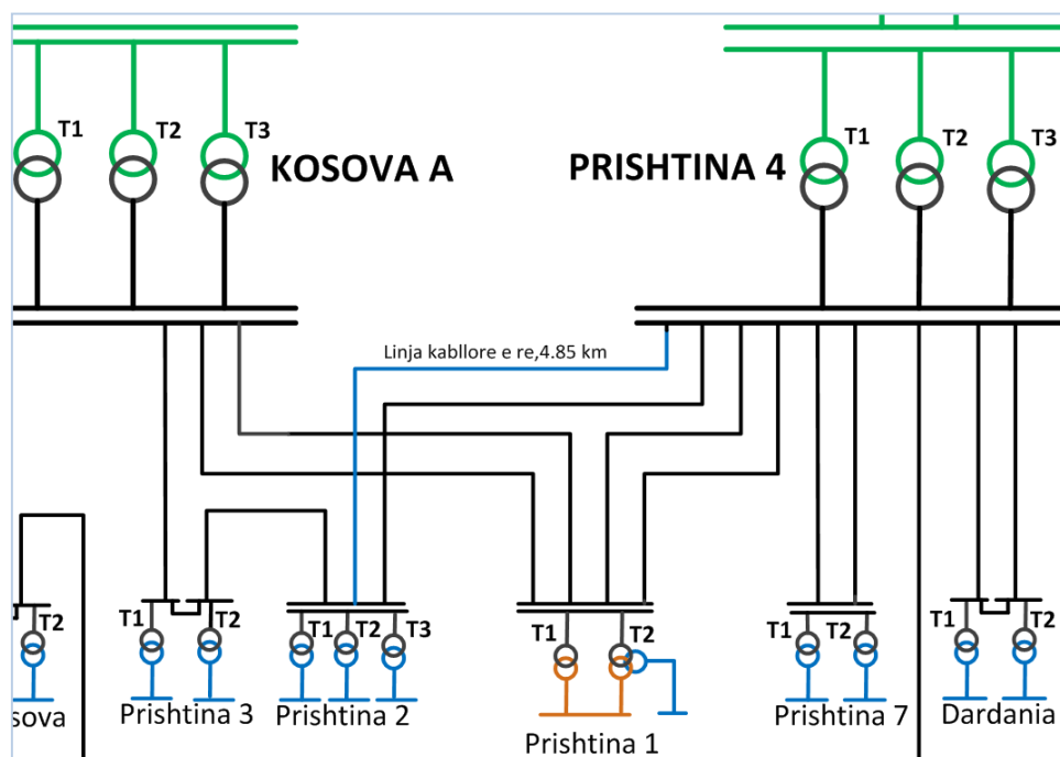
Figura 5-21. Skema njëpolare e lidhjes së linjës së re kabllore 110 kV NS Prishtina 4-NS Prishtina 2
