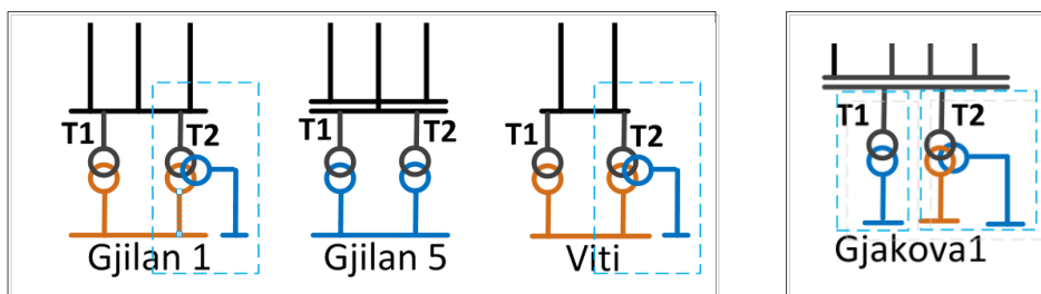
Figura 5-4. Zëvendësimi i transformatorëve në NS Viti, NS Gjilani 1 dhe NS Gjakoja 1, me transformator të ri
