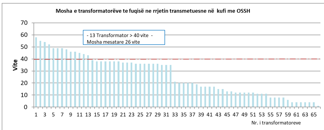
Figura 2-4. Mosha aktuale e transformatorëve të fuqisë në operim në rrjetin e transmetimit.
