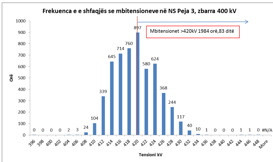
Figura 5-30. Frekuenca e shfaqjes së mbitensioneve ne zbarrat 400 kV ne NS Peja 3.
