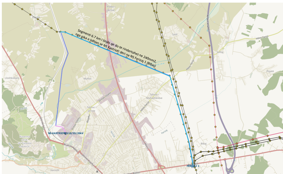
Figura 5-22. Shtirja gjeografike e projektit për ri-ndërtimin e segmentit të linjës NS Kastrioti-NS Ferizaj 1 (nga Pika e lidhjes deri te NS Ferizaj 1)
