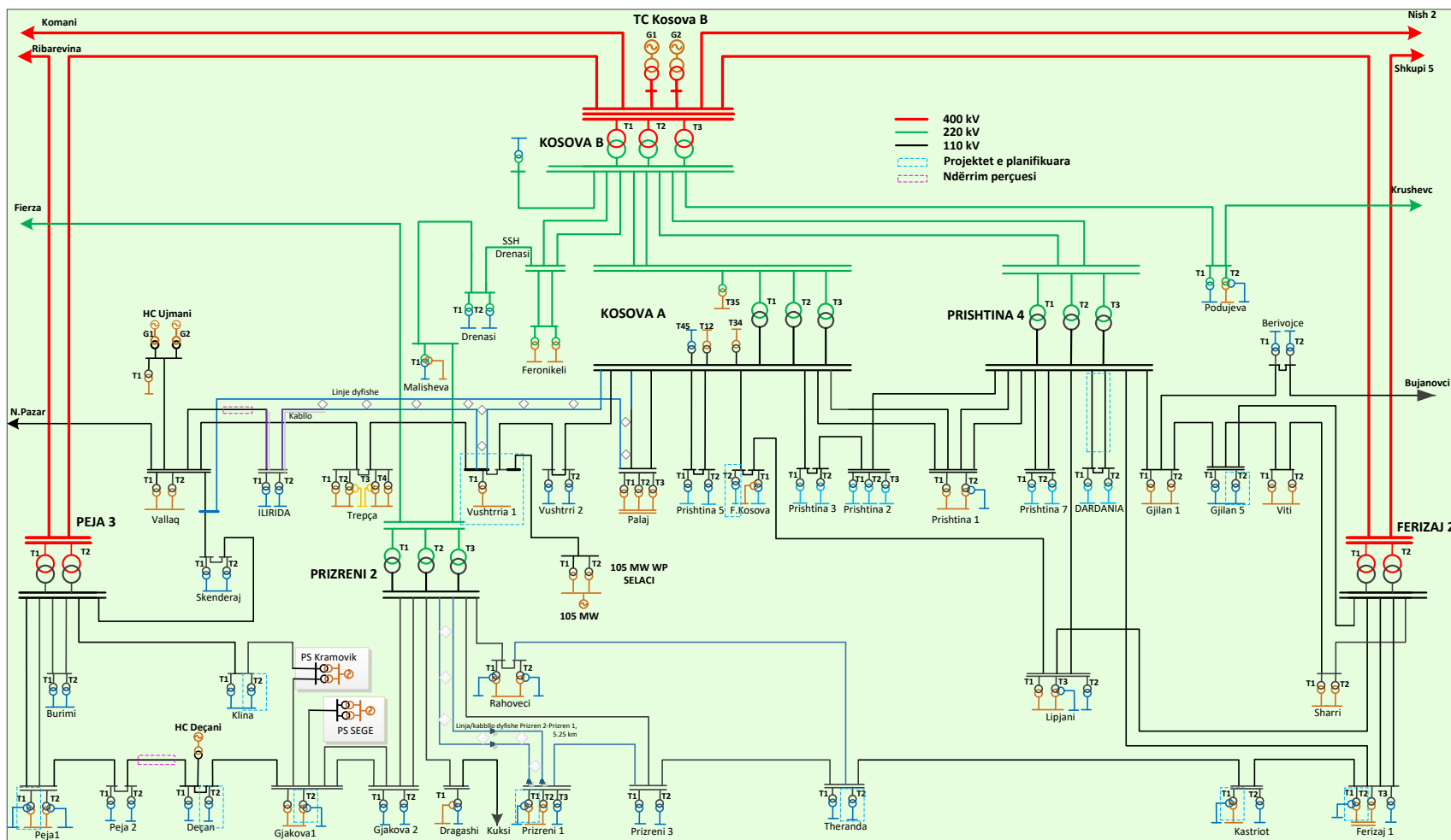
Skema njëpolare e SEE të Republikës së Kosovës - 2028
