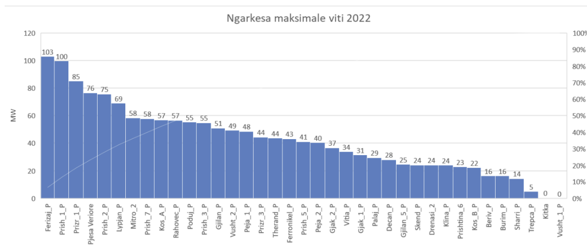
Figura 3-8 Rangimi i nënstacioneve të KOSTT ne kufi me KEDS sipas ngarkesës (2022)
