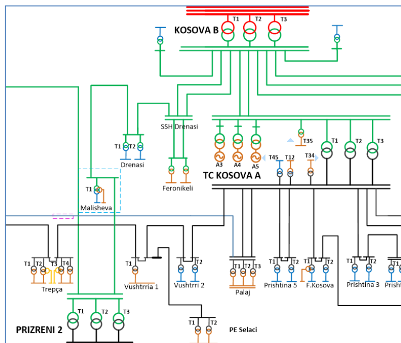
Figura 5-6 Konfiguracioni njëpolar i lidhjes së NS Malisheva ne rrjetin 220 kV Përfitimet e pritshme nga ky projekt janë:
