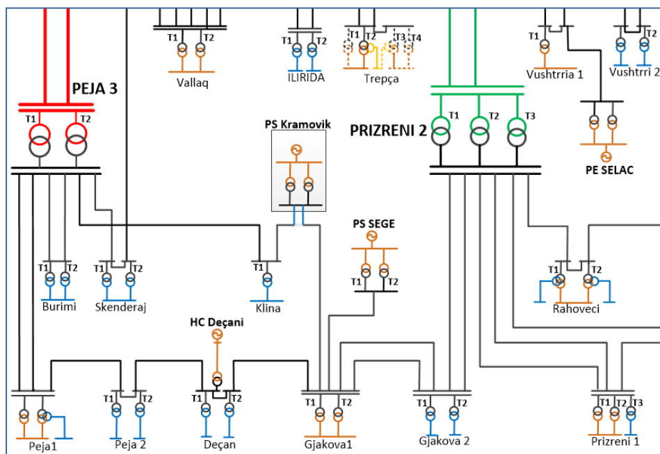
Figura 5-12. Skema njëfazore e kyçës së PS Kramovik në linjën 110 kV NS Klina- NS Gjakova 1
