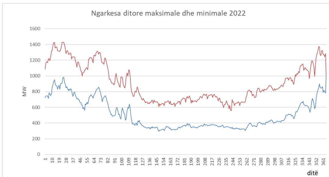
Figura 3-4 Diagrami i ngarkesës maksimale ditore dhe minimale ditore për vitin 2022
