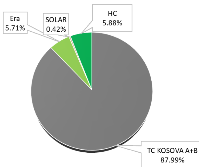
Figura 4-1 Pjesëmarrja e prodhimit të gjenerimit sipas teknologjive në vitin 2022
