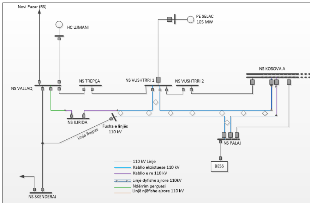
Figura 5-16 Skema njepolare e Projektit të Rivitalizimit të linjës NS Kosova A- NS Palaj- NS Ilirida-NS Vallaq
