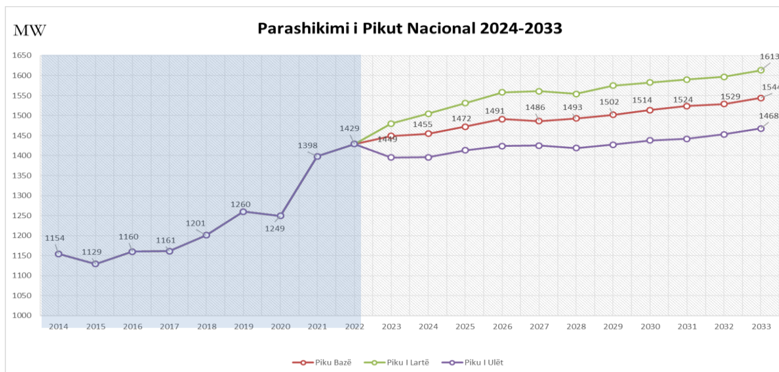
Figura. 3-10. Skenarët e zhvillimit të ngarkesës maksimale vjetore ne 10 vitet e ardhshme
