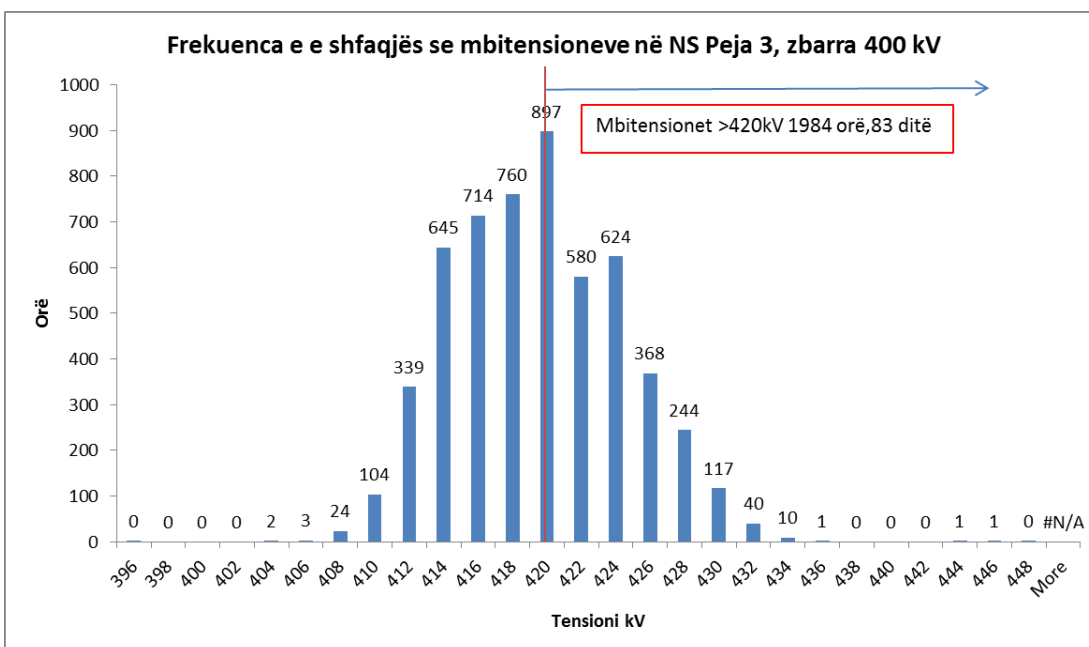
Figura 5-20. Frekuenca e shfaqjes së mbitensioneve në zbarrat 400 kV në NS Peja 3.
