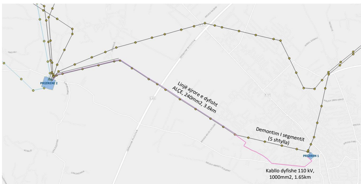
Figura 5-19 . Projekti linja dyfishte linjë/kabllo 110 kV NS Prizren 1- NS Prizren 2
