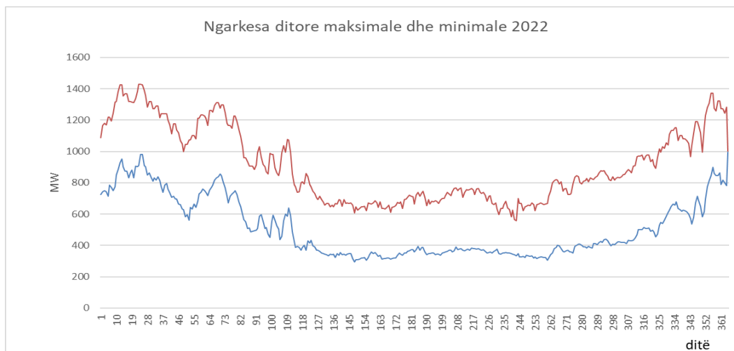
Figura 3-4 Diagrami i ngarkesës maksimale ditore dhe minimale ditore për vitin 2022
