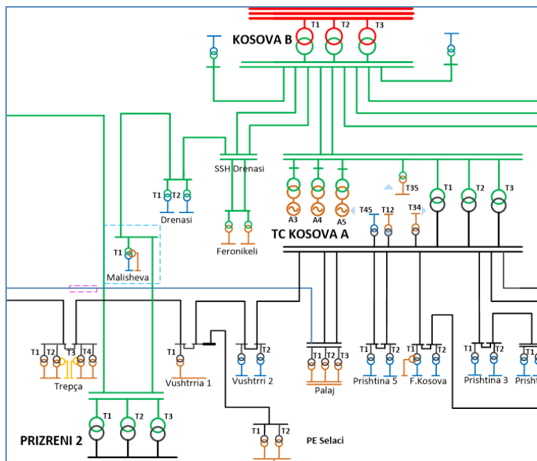
Figura 5-6 Konfiguracioni njëpolar i lidhjes së NS Malisheva në rrjetin 220 kV
