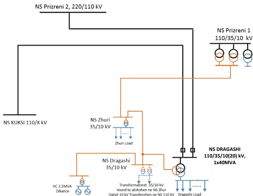
Figura 5-8 . Konfiguracioni i rrjetit të projektit: NS Dragashi dhe linja interkonektive 110 kV me NS Kukës.
