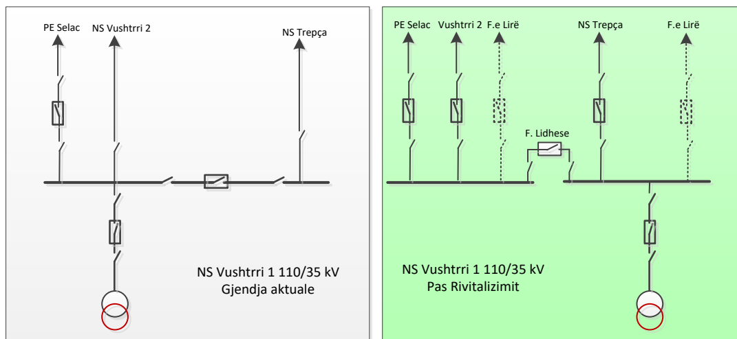
Figura 5-4 Skema aktuale e NS Vushtrri 1 dhe skema e propozuar e Rivitalizimit
