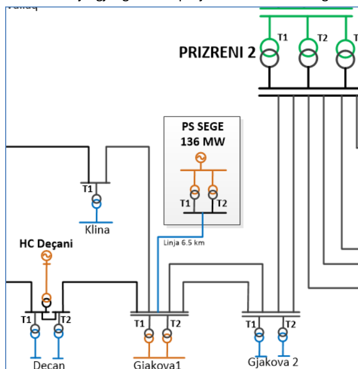
Figura 5-10. Konfiguroni i rjetit te projektit: PS SEGE
