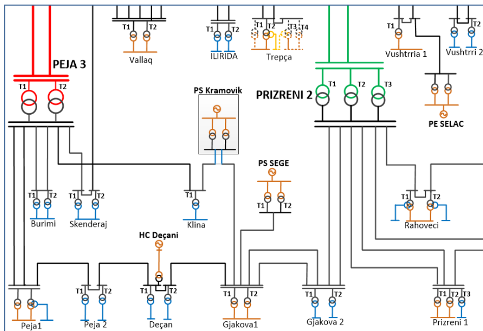
Figura 5-12. Skema njëfazore e kyçjes së PS Kramovik në linjën 110 kV NS Klina- NS Gjakova 1
