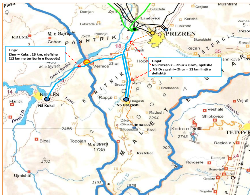
Figura 5-7 . Projekti i NS Dragashit dhe linjës 110 kV me NS Kukës.
