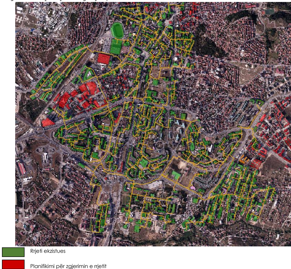
Figura 1. Shtrirja e rrjetit të ngrohjes qendrore të NP"Termokos"Sh.A në Prishtinë
