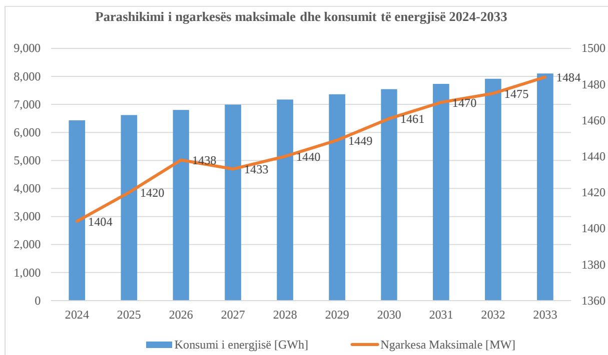
Figura 9. Parashikimi i ngarkesës maksimale dhe konsumit të energjisë për periudhën 2024-2033
