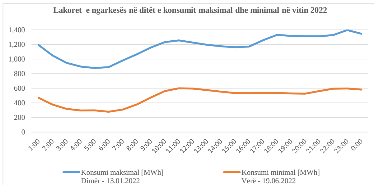
Figura 8. Lakoret e ngarkesës për ditët maksimale të dimrit dhe ato minimale të verës në vitin 2022
