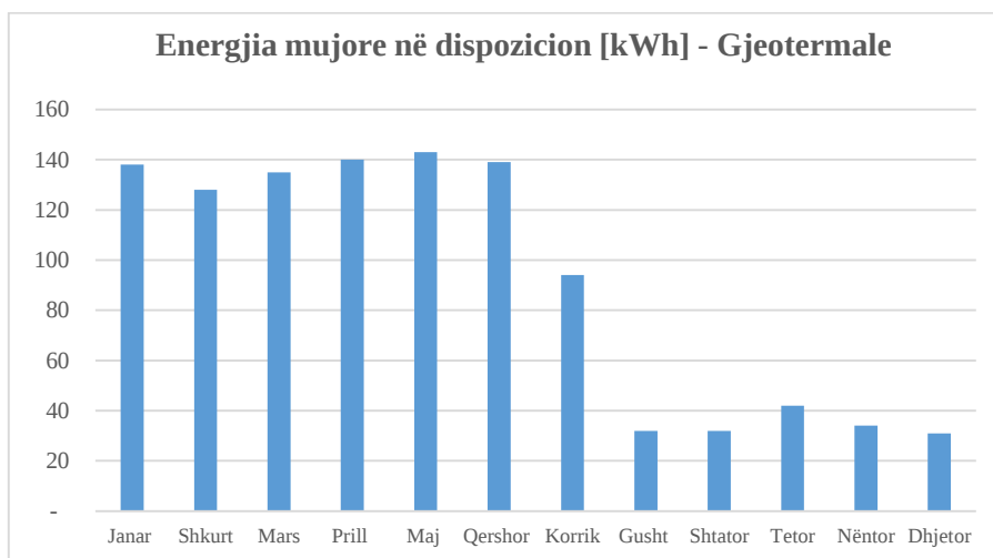
Figura 4. Energjia mujore në dispozicion [kWh] - Gjeotermale
