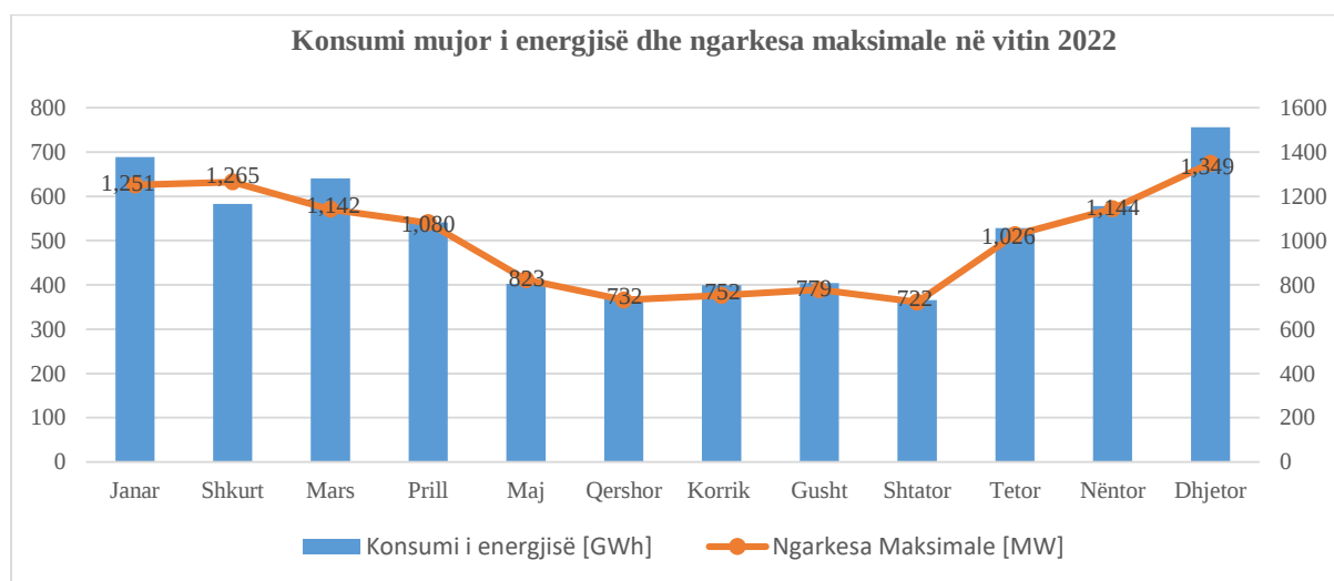
Figura 7. Konsumi mujor dhe ngarkesa maksimale në vitin 2022
