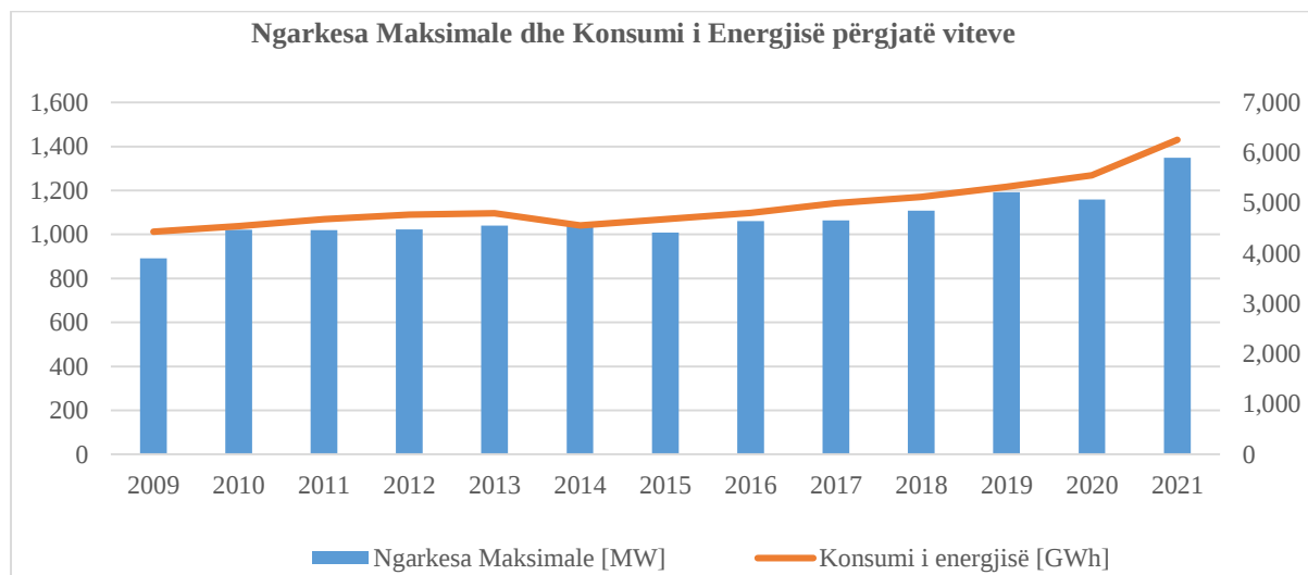
Figura 6. Konsumi vjetor i energjisë elektrike dhe ngarkesa maksimale gjatë viteve 2010-2022
