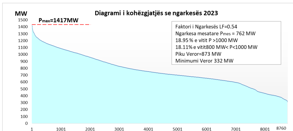
Figura 3-2 Lakorja e kohëzgjatjes së ngarkesës për vitin 2023
