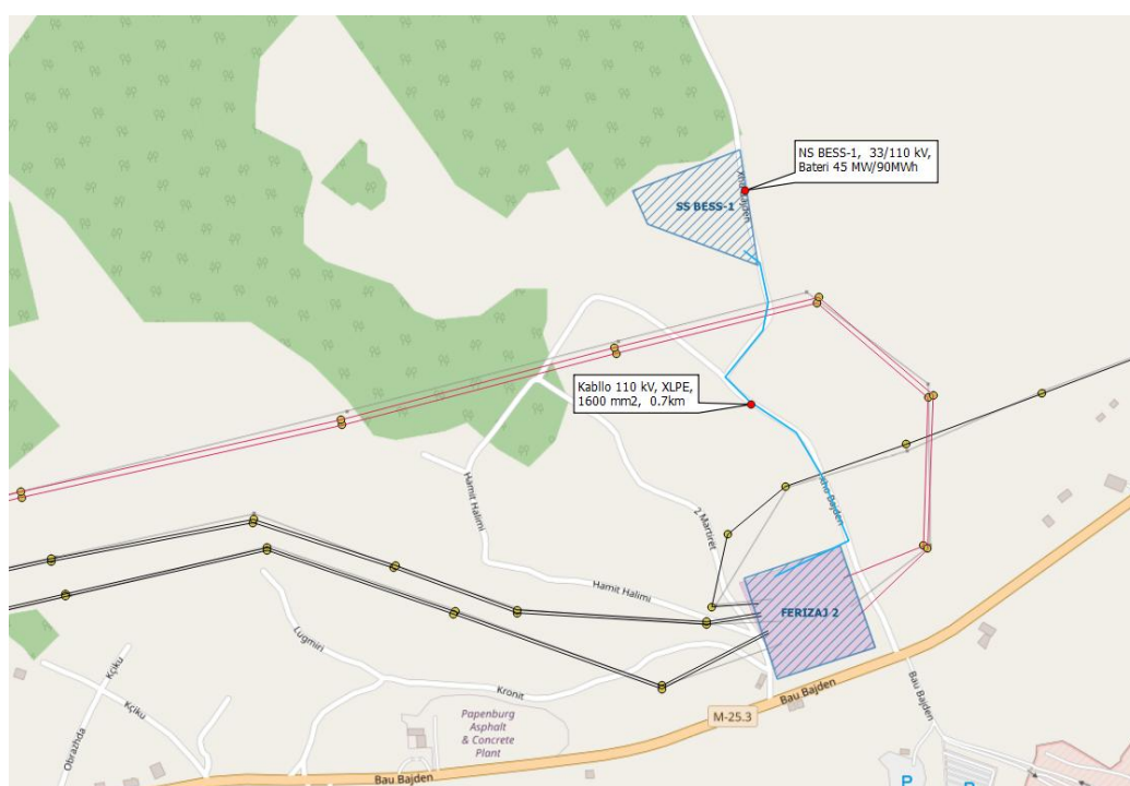
Figura 5-20. Shtrirja gjeografike e projektit BESS 1 (Bateria Akumuluese 45 MW/90MWh)
