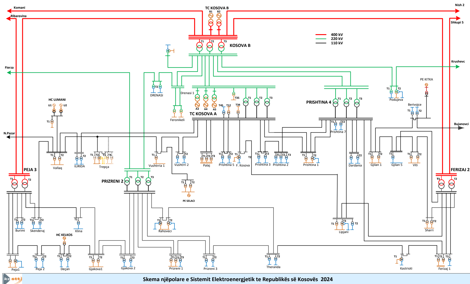
Figura 7-8 Skema njëpolare e SEE të Kosovës sipas topologjisë së rrjetit 2024
