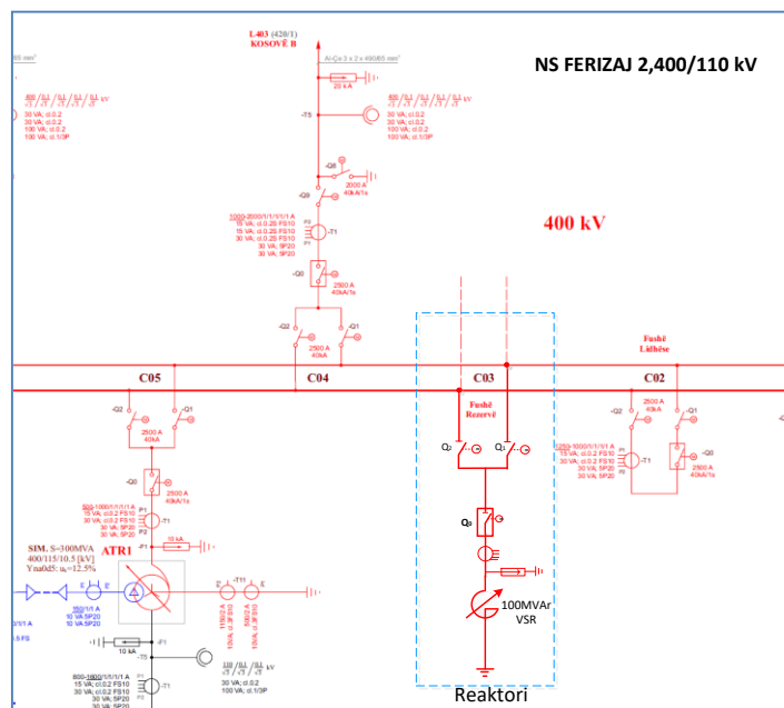
Figura 5-36. Skema njëpolare e vendosjes së reaktorit 100MVAR ne NS Ferizaj 2
