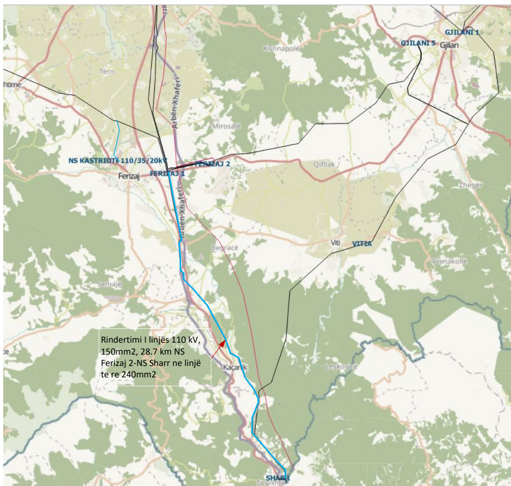
Figura 5-30. Shtrirja gjeografike e projektit: ri-ndërtimi i linjës 110 kV NS Ferizaj 2-NS Sharr duke filluar nga NS Bibaj deri ne NS Sharr
