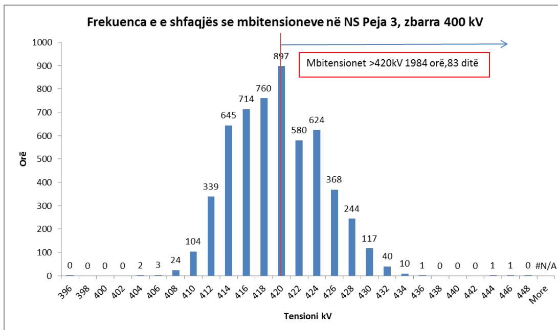
Figura 5-35. Frekuenca e shfaqjes së mbitensioneve ne zbarrat 400 kV ne NS Peja 3.
