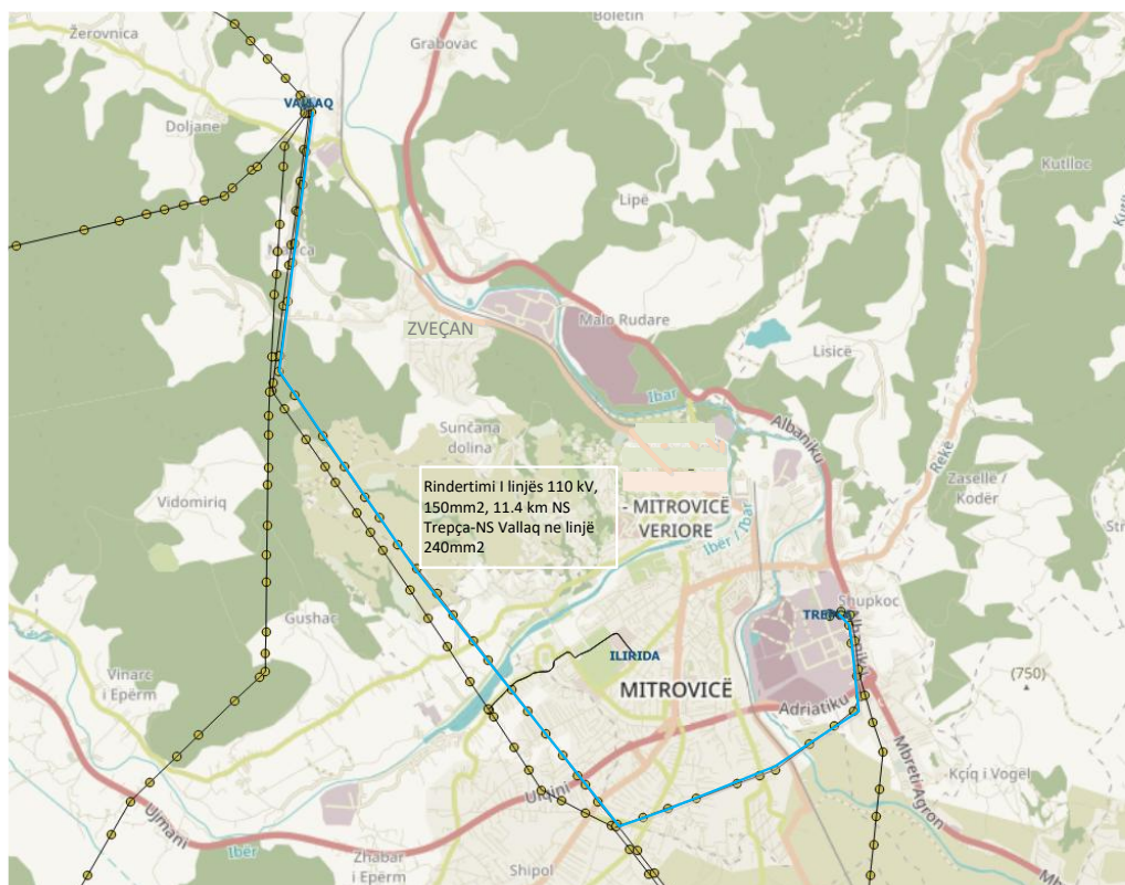
Figura 5-31 Projekti i Rivitalizimit të linjës Trepça-Vallaq
