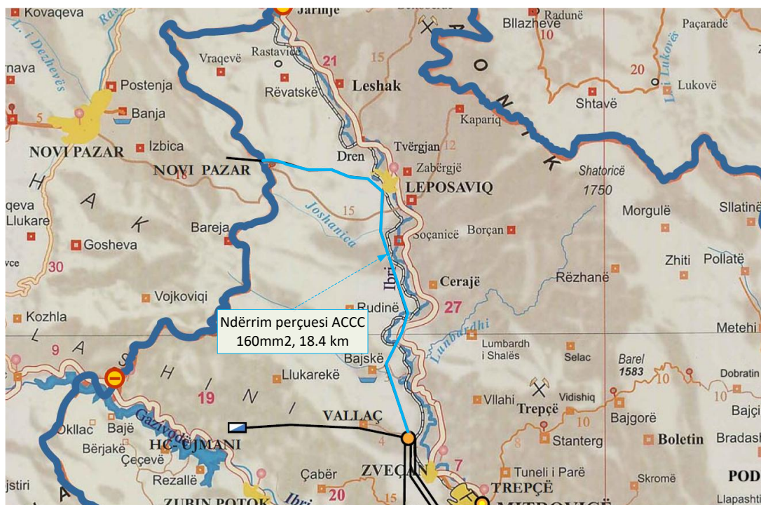
Figura 5-34 Projekti i ri-vitalizimit të linjës ndërkufitare 110 kV Vallaq-N Pazar
