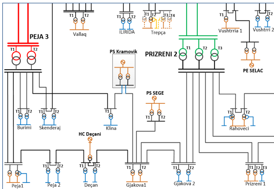
Figura 5-19. Skema njëfazore e kyçjes së PS Kramovik në linjën 110 kV NS Klina- NS Gjakova 1
