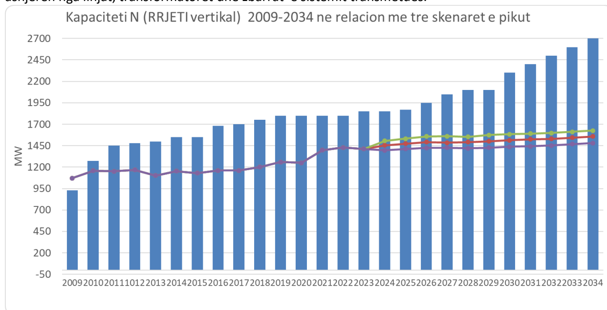
Figura 7-4. Zhvillimi i kapaciteteve të brendshme (vertikal) të rrjetit në relacion me zhvillimin e ngarkesës për 10 vitet e ardhshme
