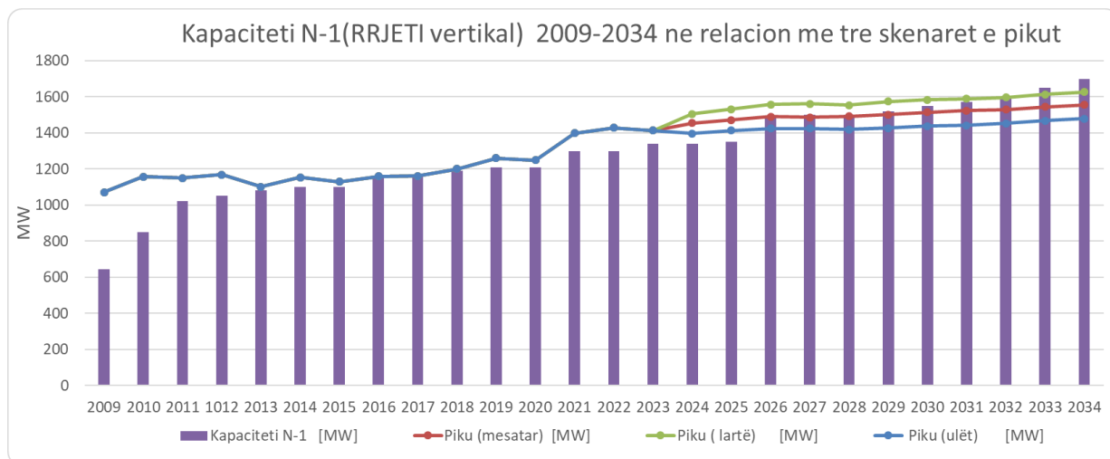
Figura 7-6. Zhvillimi i kapaciteteve N-1 të rrjetit vertikal të transmetimit 2009-2034
