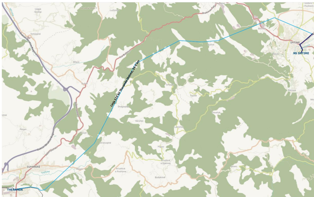
Figura 5-32 Projekti i Rivitalizimit të linjës NS Theranda-NS Shtime (pjesa me përçues 150mm 2 )
