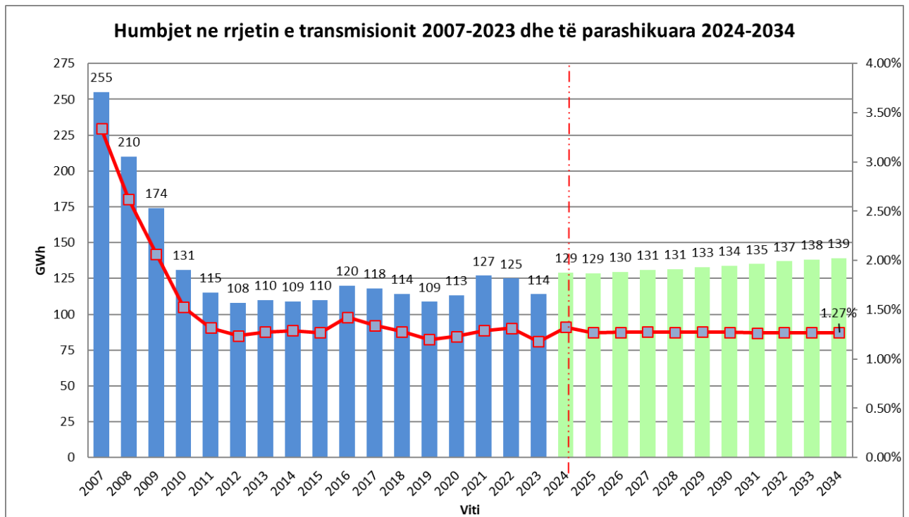
Figura 7-7. Humbjet e energjisë aktive ne rrjetin e transmetimit 2007-2023 dhe parashikimi 2024-2034
