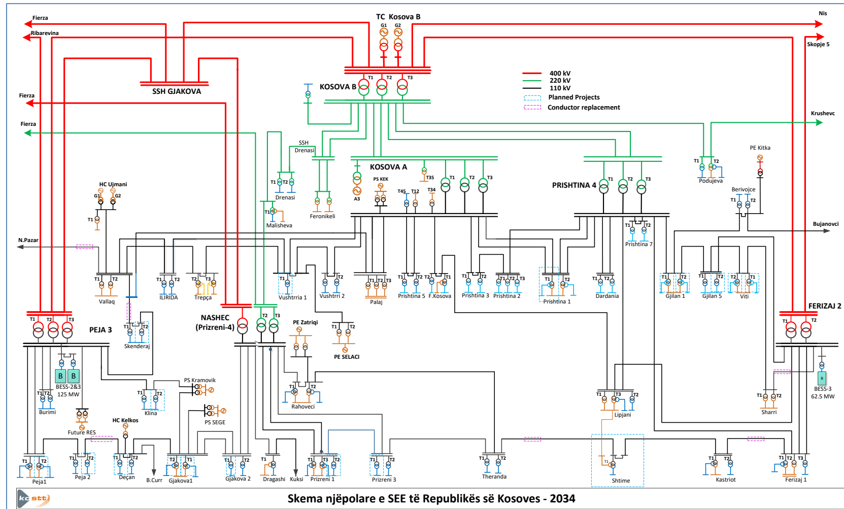
Figura 7-10 Skema njëpolare e SEE të Kosovës sipas topologjisë së rrjetit 2034
