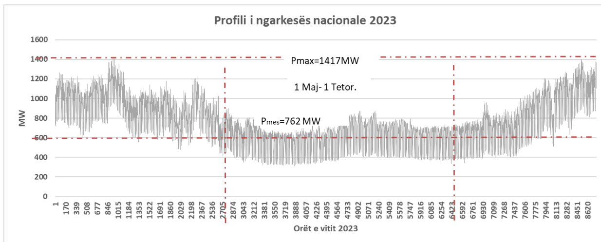
Figura 3-3 Diagrami orë për orë i ngarkesës vjetore e realizuar gjatë vitit 2023
