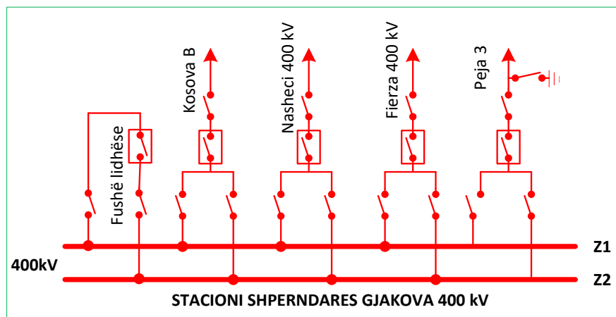
Figura 5-39. Skema njëpolare e stacionit shpërndarës SSH GJAKOVA 400 kV
