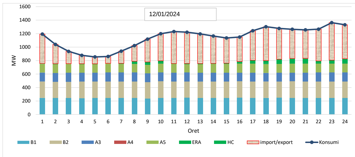
Figura 3-6 Diagrami i ngarkesës ditore dhe prodhimi për pikën referencë (Janar 2024)
