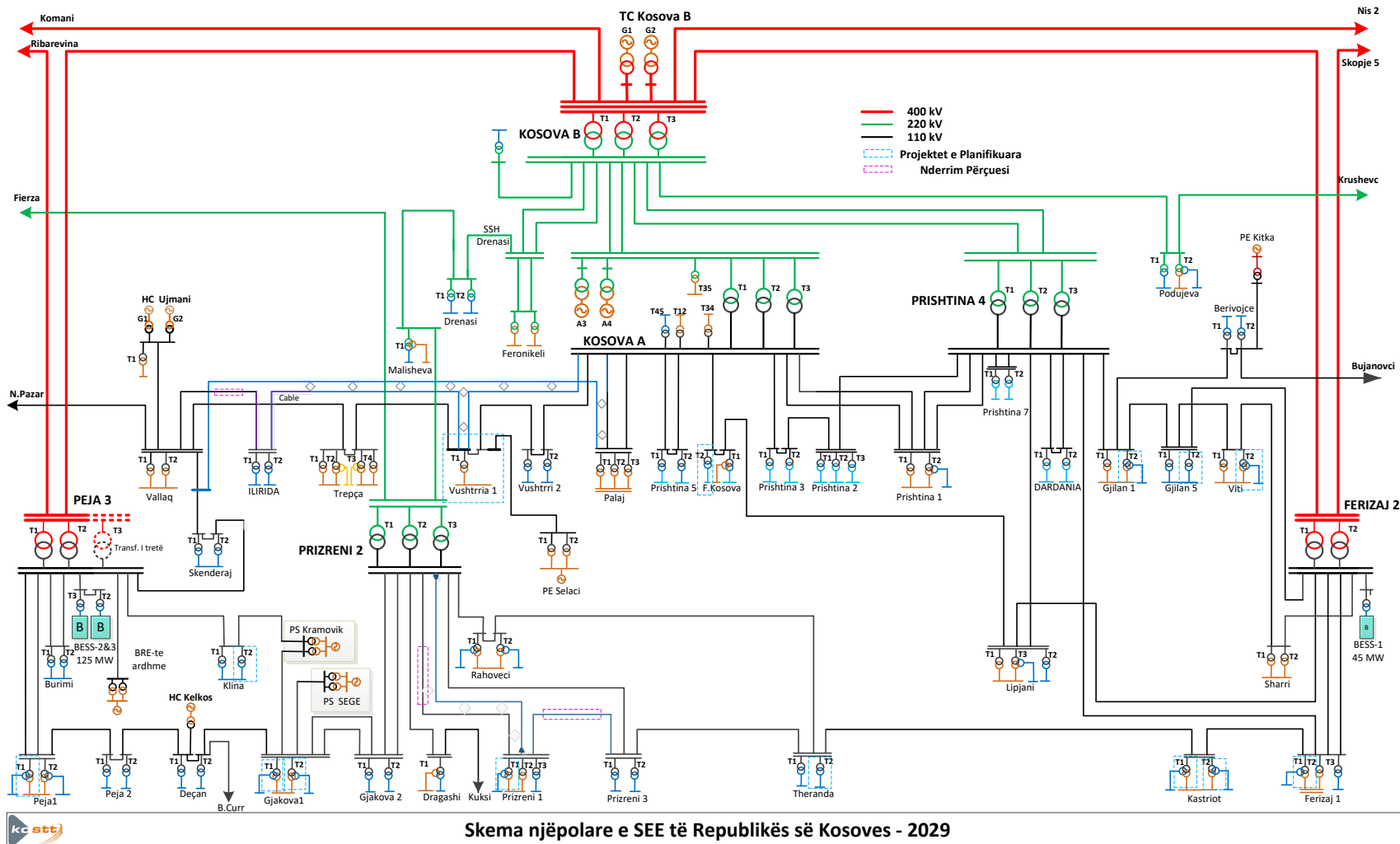
Figura 7-9 Skema njëpolare e SEE të Kosovës sipas topologjisë së rrjetit 2029
