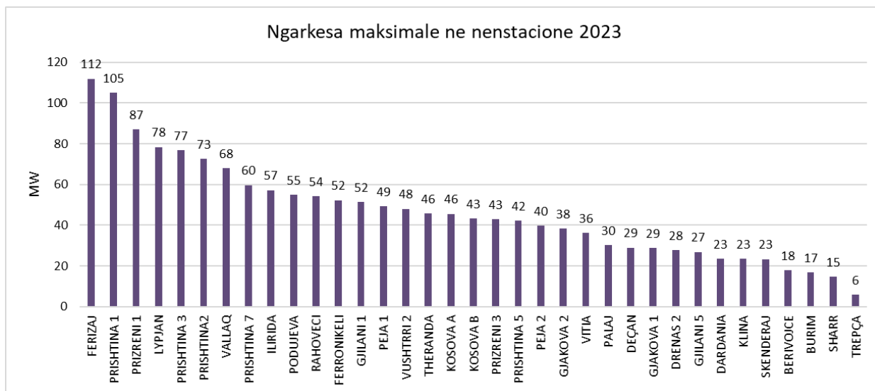
Figura 3-8 Rangimi i nënstacioneve të KOSTT ne kufi me KEDS sipas ngarkesës(2023)
