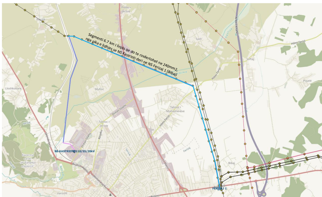
Figura 5-27. Shtrirja gjeografike e projektit për ri-ndërtimin e segmentit të linjës NS Kastrioti-NS Ferizaj 1 (nga Pika e lidhjes deri te NS Ferizaj 1)
