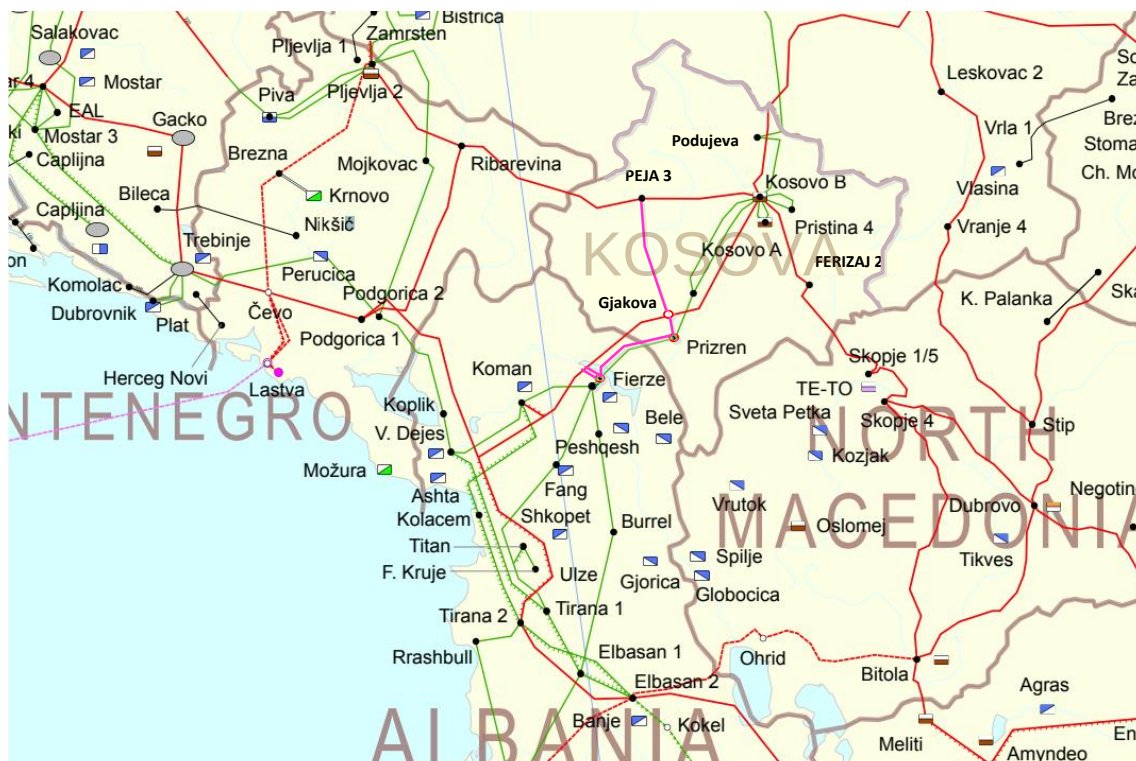
Figura 5-38 Shtrirja gjeografike e projektit te unazës 400kV SSH Gjakova-NS Nashec- NS Peja 3 (Harta e ENTSO-E)
