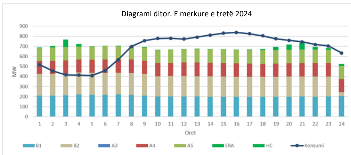
Figura 3-7 Diagrami i ngarkesës ditore dhe prodhimi për pikën referencë (e mërkturë e 3-të, Korrik 2024)
