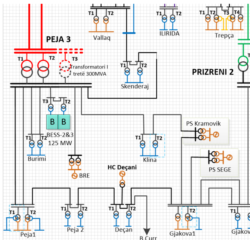
Figura 5-23. Skema njëpolare e projektit BESS -2&3 (Bateria Akumuluese 2x62.5MW/250 MWh)
