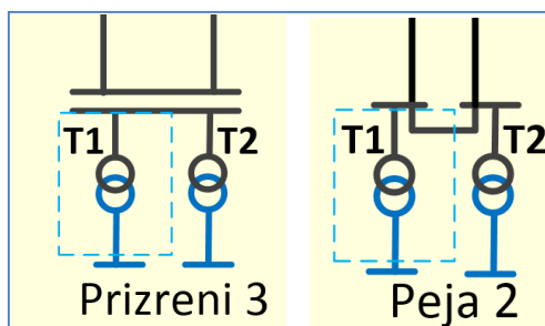
Figura 5-8. Zëvendësimi i transformatorit TR-1 në NS Prizren 3 dhe TR-1 në NS Peja 2
