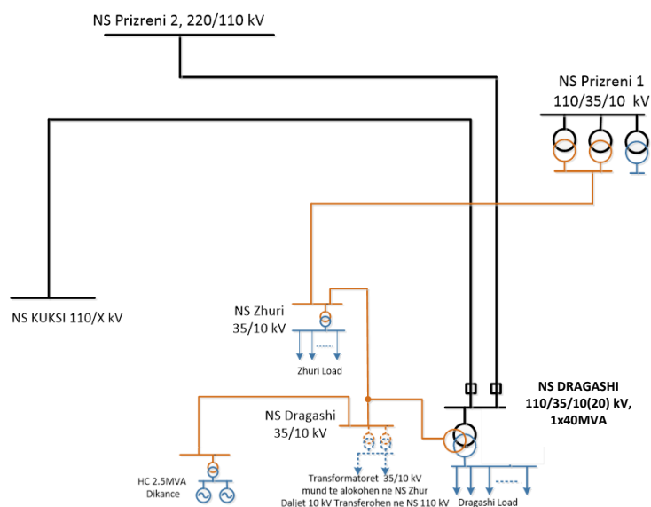
Figura 5-13 . Konfiguracioni i rrjetit të projektit: NS Dragashi dhe linja interkonektive 110 kV me NS Kukës.
