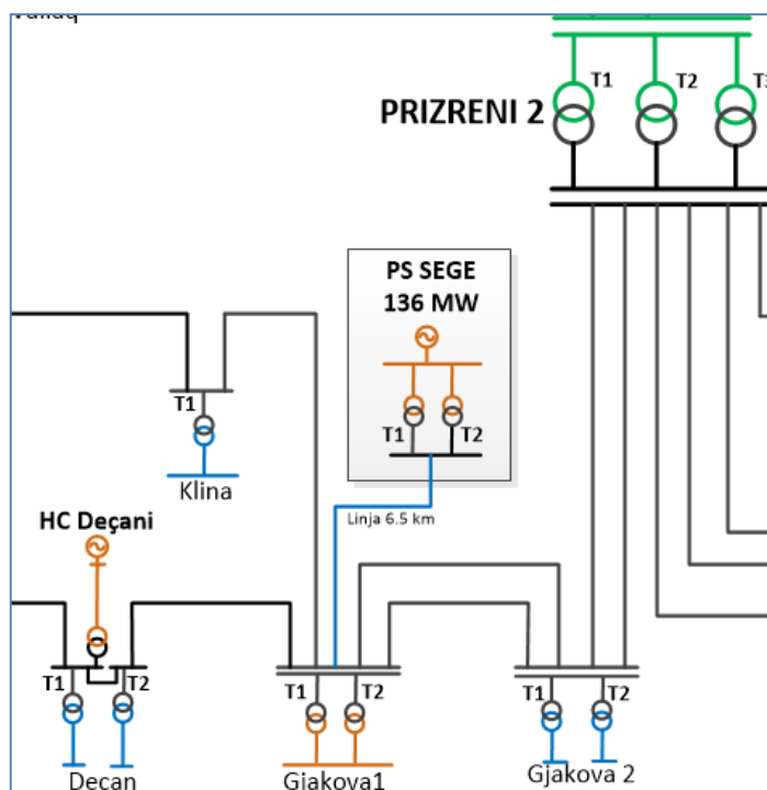
Figura 5-17. Konfiguracioni i rrjetit te projektit: PS SEGE
