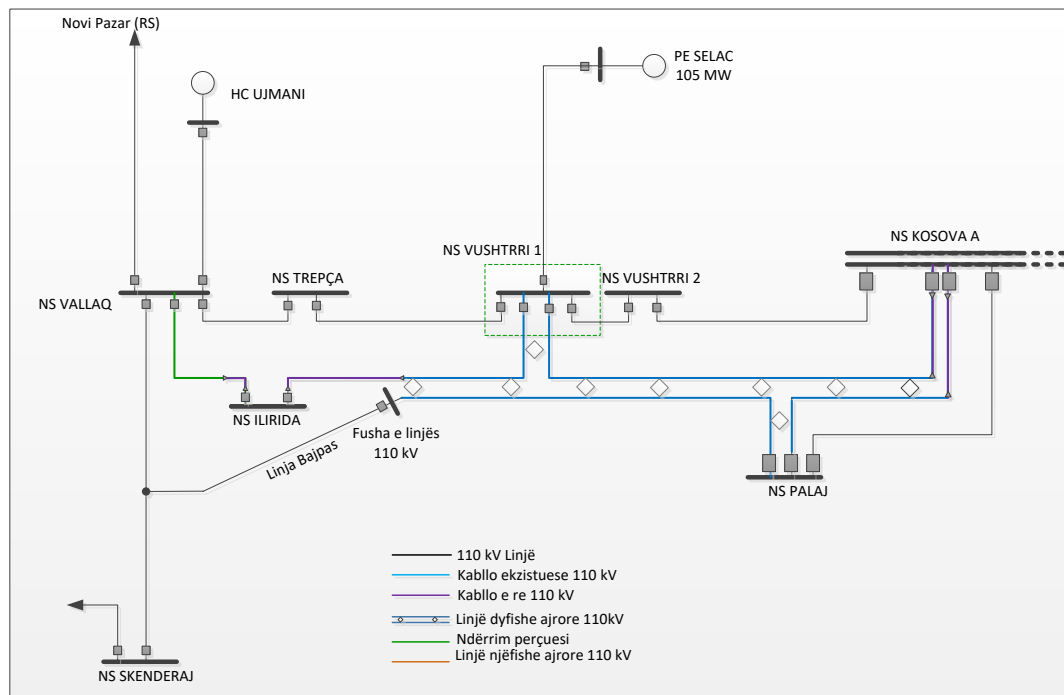
Figura 5-25 Skema njepolare e Projektit e Rivitalizimit te linjës NS Kosova A- NS Palaj- NS Ilirida-NS Vallaq
