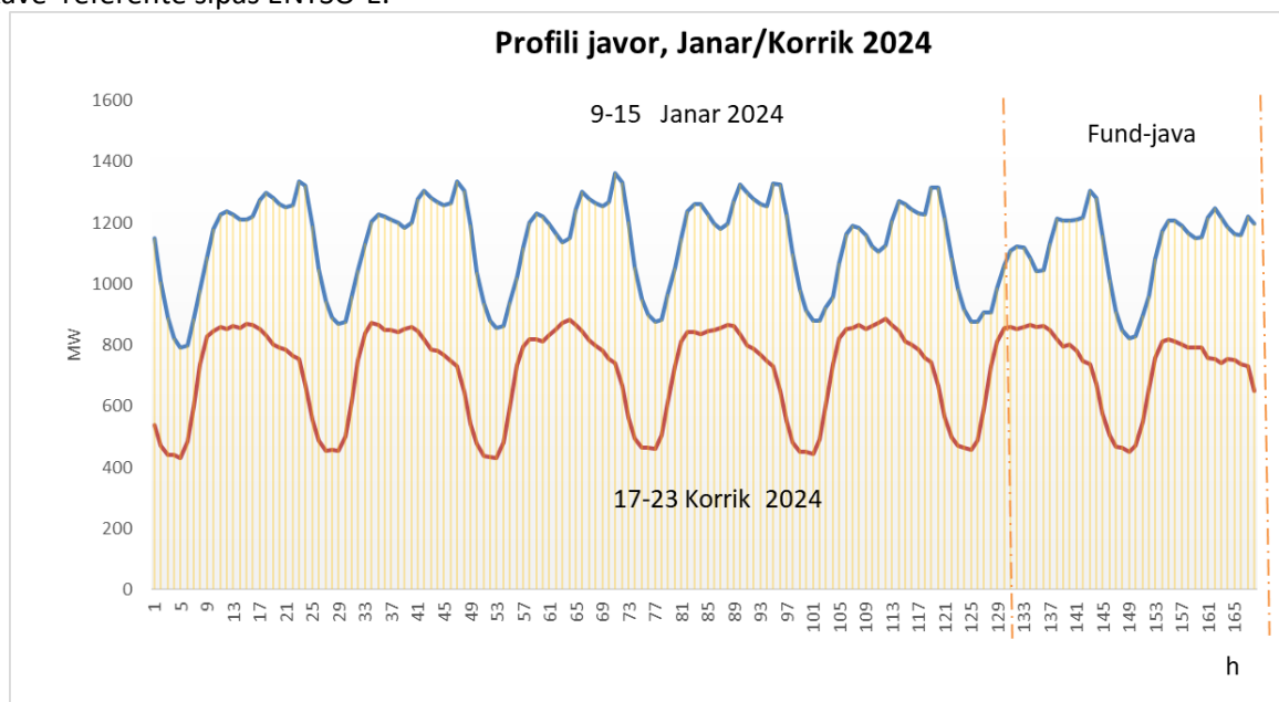
Figura 3-5 Diagrami tipik javor i janarit dhe korrikut 2024
