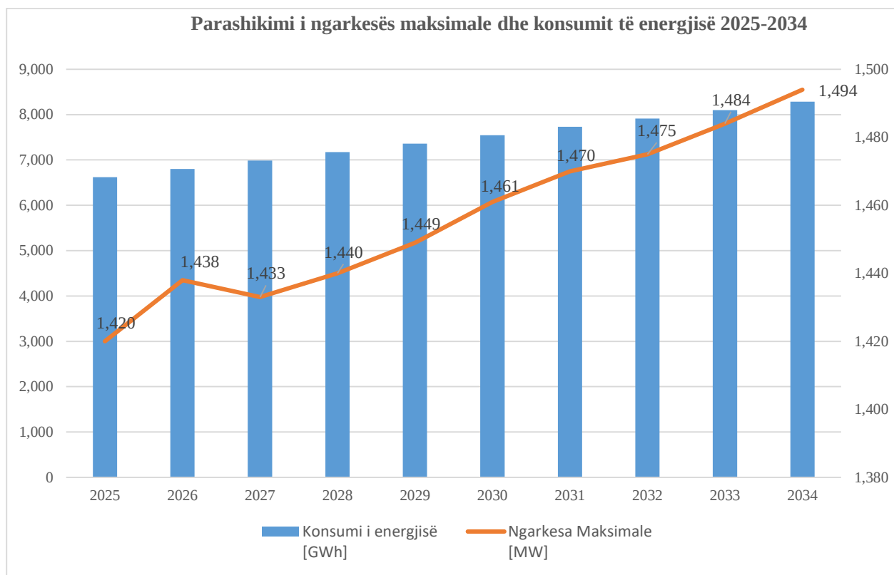
Figura 9. Parashikimi i ngarkesës maksimale dhe konsumit të energjisë për për periudhën 2026-2035
