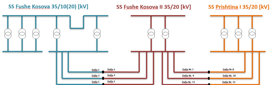
Figura 10. Lidhja unazore mes NS Fushë Kosova, NS Fushë Kosova II dhe NS Prishtina I
