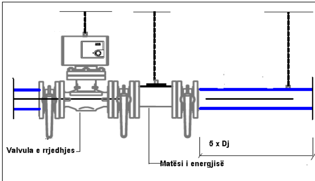
Fig. 2. Skema e matësit të energjisë dhe valvulës së rrjedhjes
