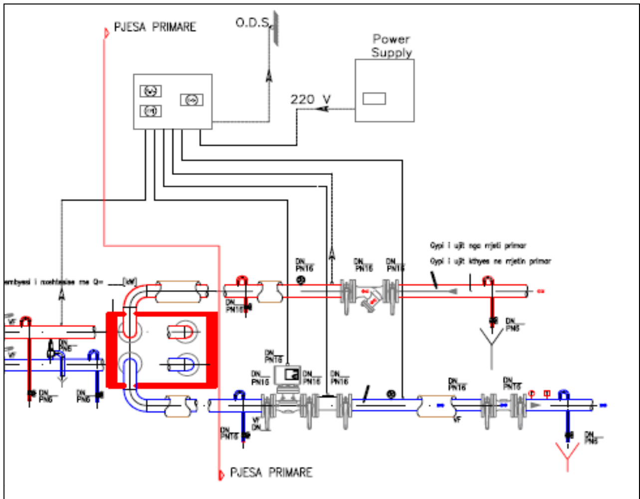
Fig. 1. Skema funksionale e nënstacionit termik – Pjesa primare Skema e lidhjes së matësit të energjisë dhe valvulës së rrjedhjes
