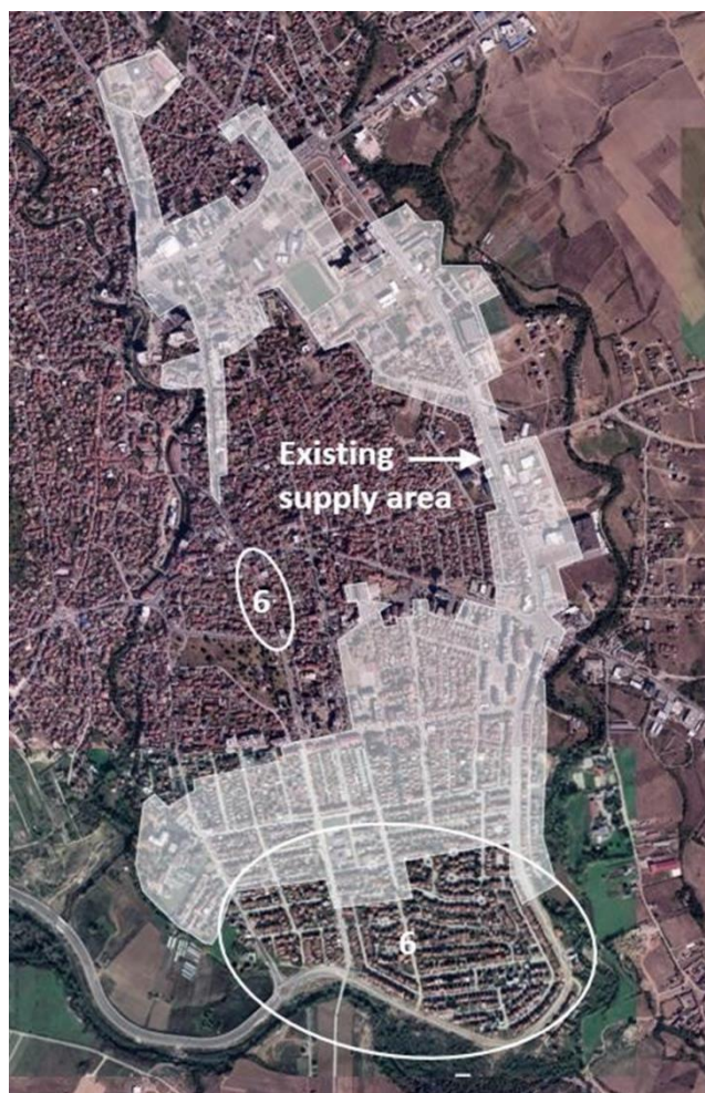
Figura 4. Zonat e zgjerimit të rrjetit të shpërndarjes, 2029 – 2036
