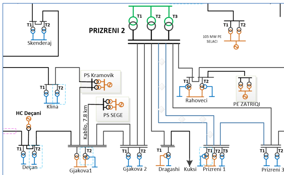
Figura 5-19. Konfiguracioni i rrjetit të projektit: PS SEGE
