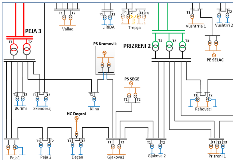
Figura 5-21. Skema njëfazore e kyçjes së PS Kramovik në linjën 110 kV NS Klina- NS Gjakova 1
