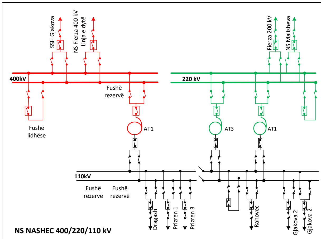
Figura 5-44. Skema njëpolare e nënstacionit NS Prizreni 2, 220/110 kV të ri-ngritur në NS Nashec, 400/220/110 kV
