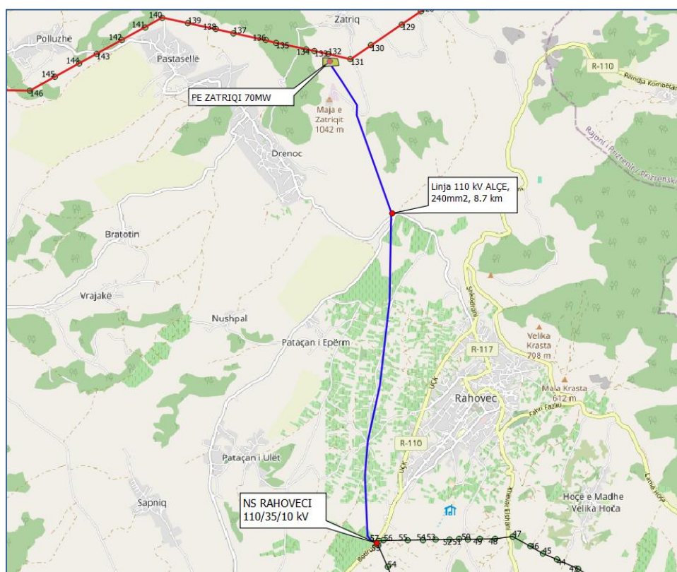
Figura 5-22. Shtrirja gjeografike e projektit Parku me Erë Zatriqi 70 MW
