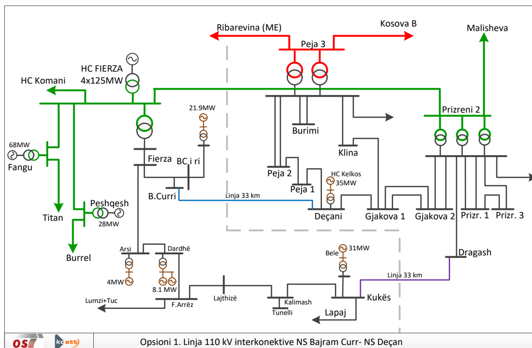
Figura 5-41. Projekti i linjës së dytë interkonektive NS Bajram Curri-NS Deçani
